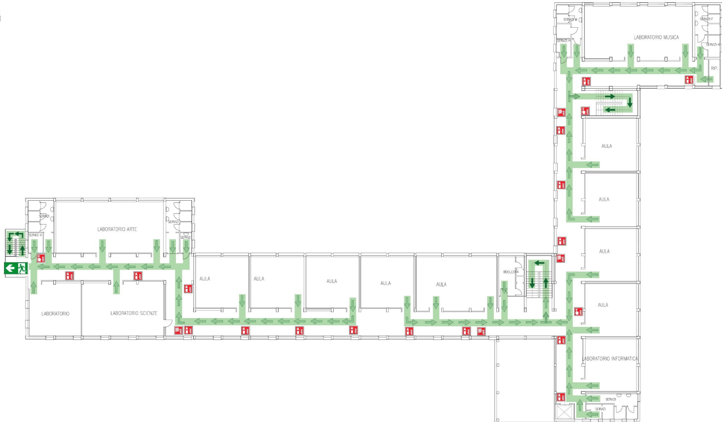
PLANIMETRIA GENERALE
